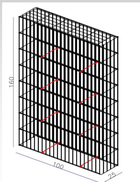
8 St. Distanzhalter
